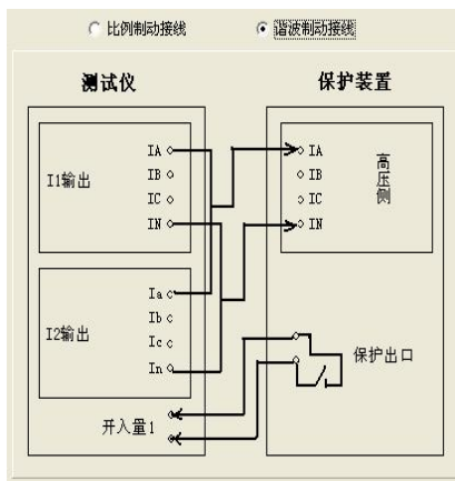
六相电流接线
