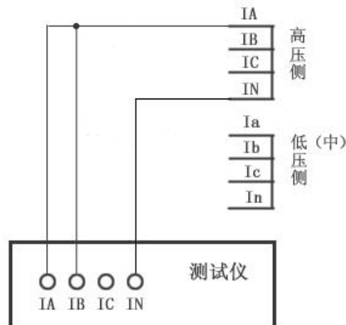
三相电流接线
